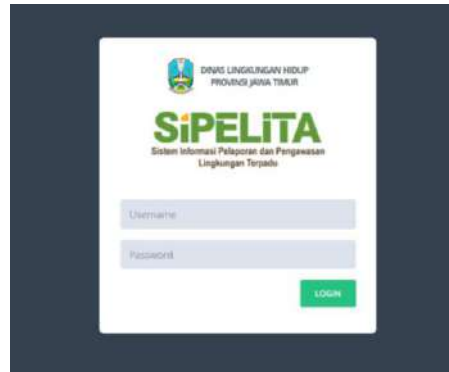
Gambar 2. 3 Aplikasi SiPelita
