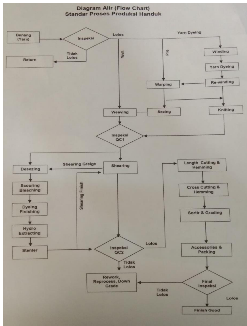
Gambar 2.3 Alur proses produksi handuk
