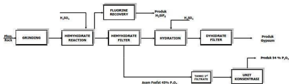
Gambar II. 2 Diagram Alir Produksi Asam Fosfat
