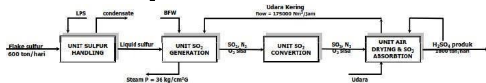
Gambar II. 1 Diagram Alir Proses Produksi Asam Sulfat
