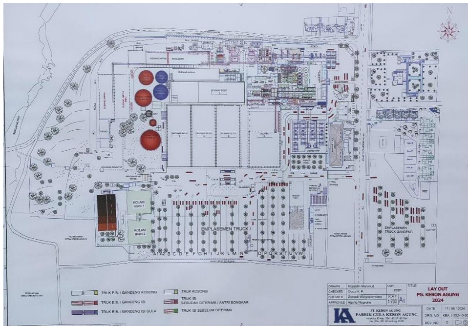
Gambar I.3 Tata Letak PG Kebon Agung Malang
