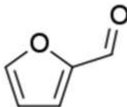
Gambar I.1 Struktur Molekul Furfural
