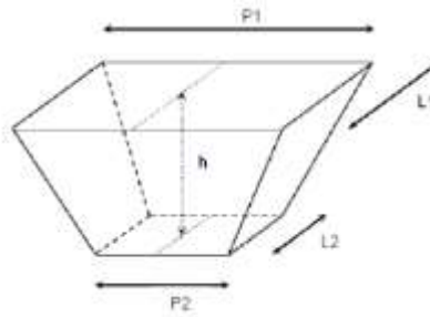
Gambar 2. 11 Sketsa Dimensi Ruang Lumpur
