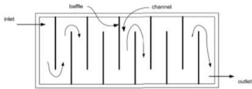
Gambar 2. 8 Pengadukan Lambat dengan Baffled Channel
