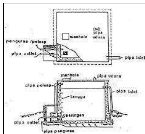
Gambar 2. 13 Reservoir Permukaan
