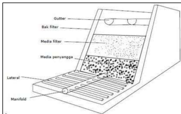
Gambar 2. 12 Bagian-Bagian Filtrasi
