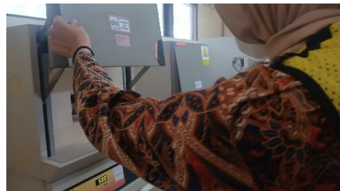
Gambar 4. Memasukkan Sampel yang telah ditimbang ke dalam Furnace
