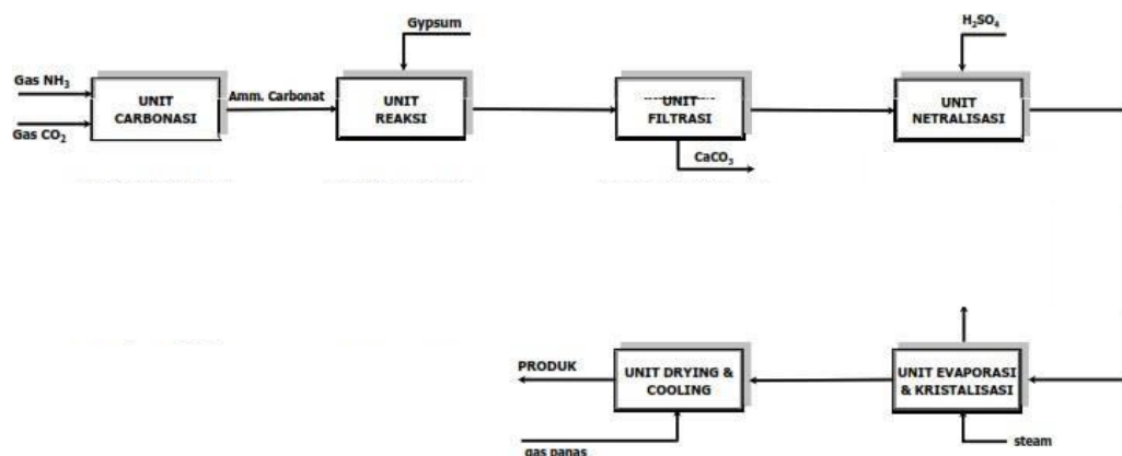
Gambar II. 3 Diagram Alir Proses Produksi Ammonium Sulfat
