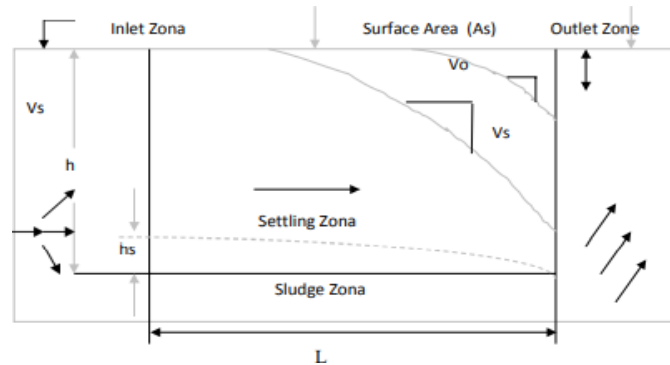
Gambar 2 9 Zona Pada Bak Sedimentasi
