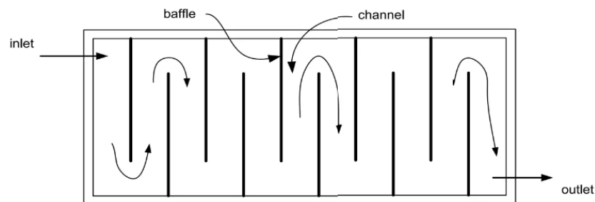
Gambar 2 8 Pengadukan Lambat dengan Baffled Channel
