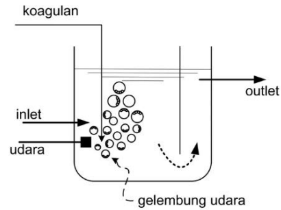
Gambar 2 6 Pengadukan Cepat Secara Pneumatis
