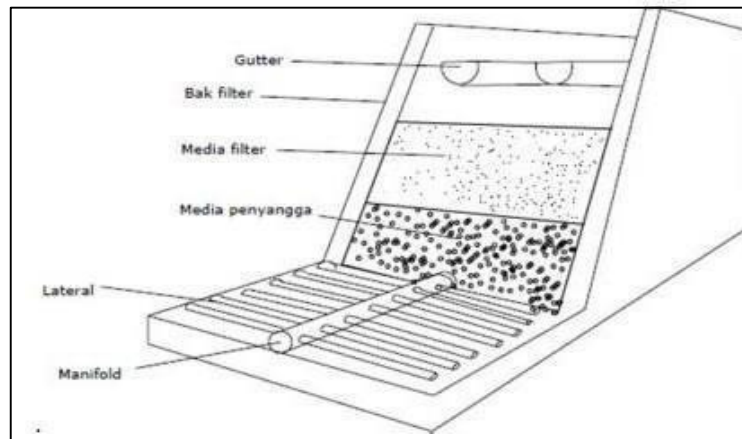
Gambar 2 12 Bagian-Bagian Filtrasi
