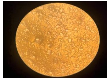
Gambar 10. Hasil mikroskop dari gula di stasiun masakan
