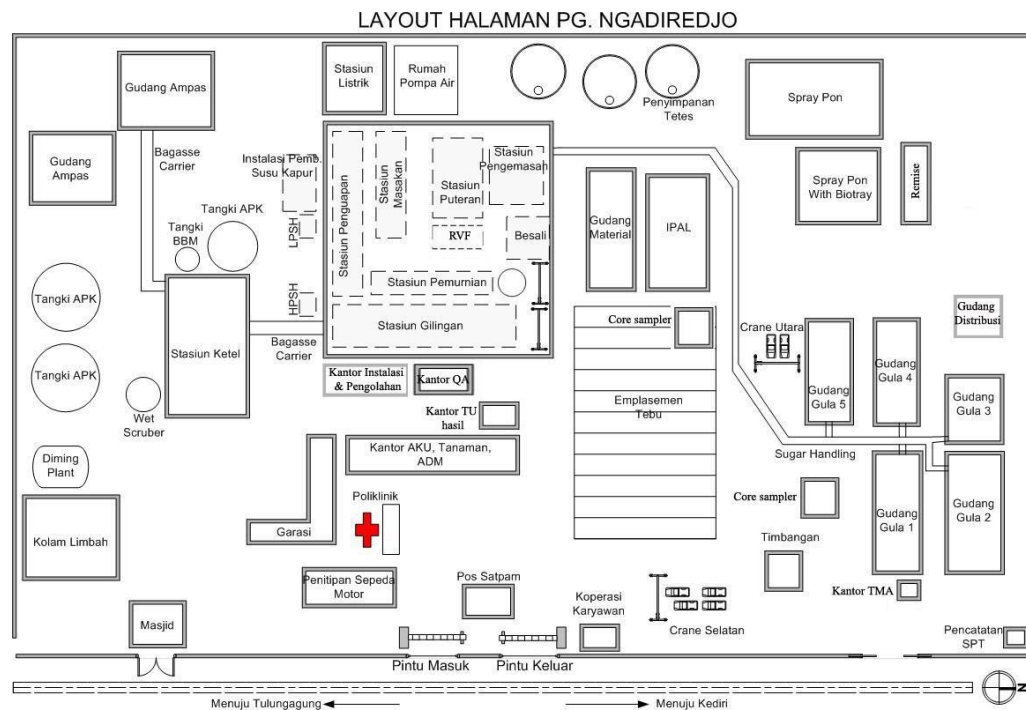
Gambar I. 5 Layout Pabrik PG. Ngadiredjo Kediri
