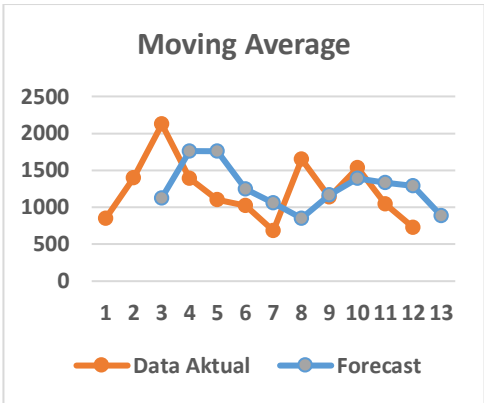
Gambar 4. Grafik perbandingan data aktual dengan forecast metode Moving Average Sumber: (Penulis, 2024)
