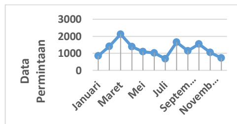
Gambar 2. Grafik Permintaan Handuk Tipe A Tahun 2024
