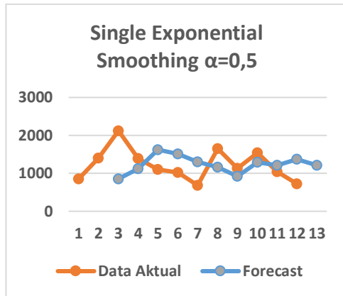
Gambar 6. Grafik perbandingan data aktual dengan forecast metode Single Exponential Smoothing \alpha=0,5 Sumber: (Penulis, 2024)
