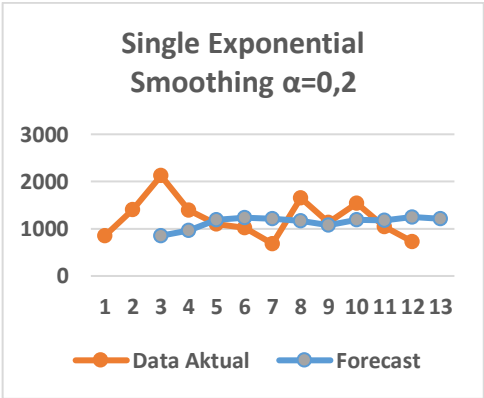
Gambar 5. Grafik perbandingan data aktual dengan forecast metode Single Exponential Smoothing \alpha=0,2 Sumber: (Penulis, 2024)
