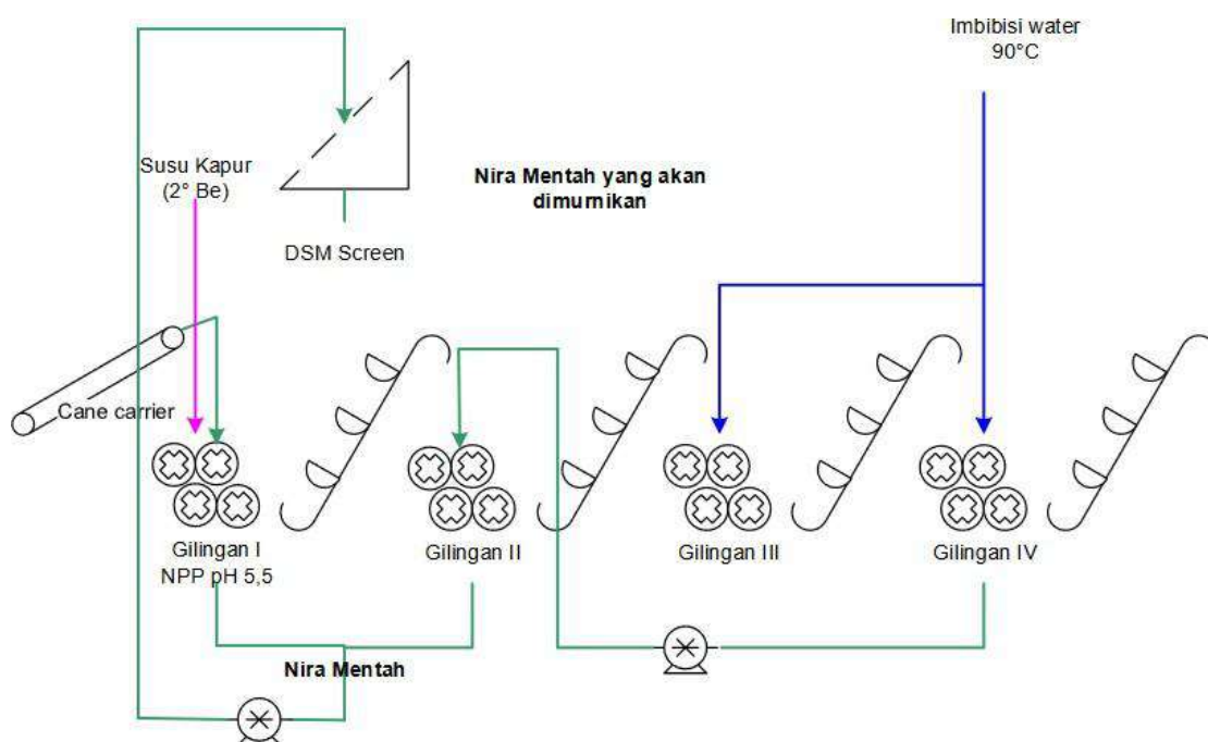
Gambar 2. 1 Gambaran Proses Stasiun Gilingan
