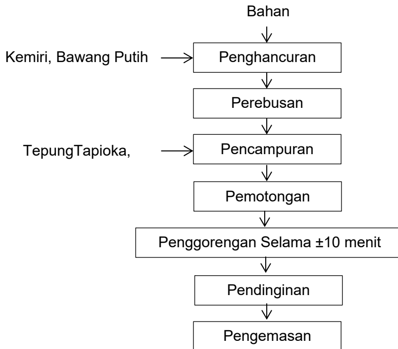
Gambar 2.9. Diagram Alir Proses Produksi Kripik Bakiak
