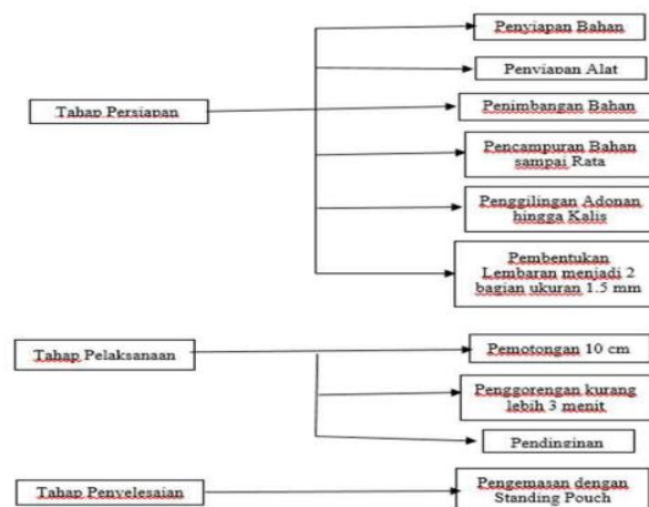
Gambar 2.8 Tahapan Proses Pembuatan Stik
