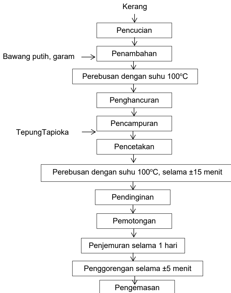
Gambar 2.11. Diagram Alir Proses Produksi Kerupuk Kerang
