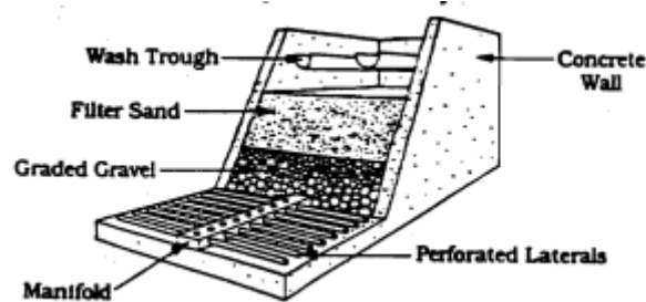
Gambar 2. 19 Bagian – bagian filter
