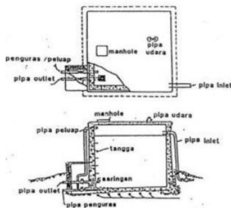
Gambar 2. 20 Reservoir Permukaan
