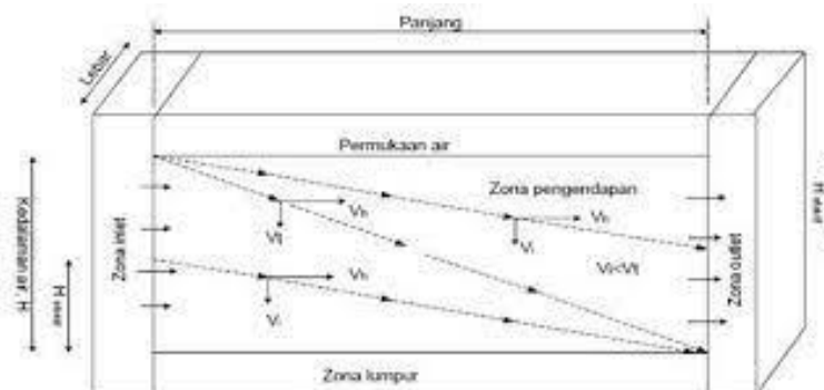
Gambar 2. 15 Zona pada Bak Sedimentasi
