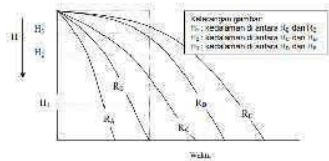
Gambar 2. 17 Grafik Isoremoval
