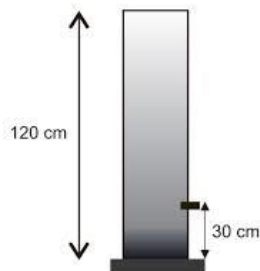
Gambar 2. 16 Kolom Test Sedimentasi Tipe II
