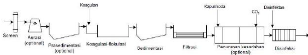
Gambar 2. 1 Skema Unit Pengolahan Air Minum
