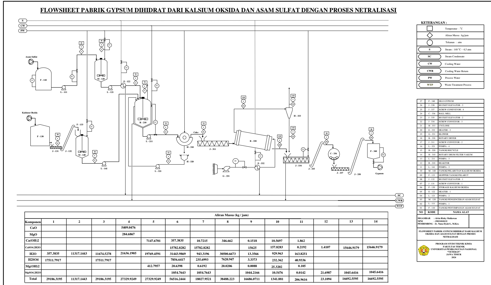
Gambar 1. Flowsheet Perencanaan Pabrik
