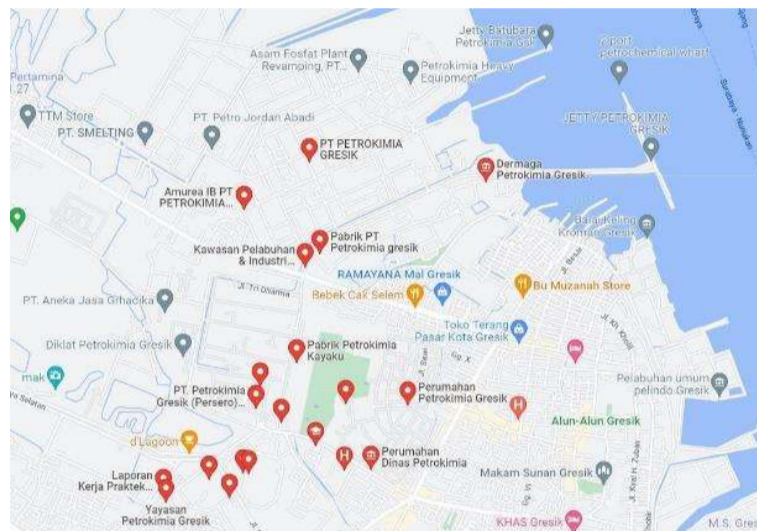
Gambar I. 2 Peta lokasi PT. Petrokimia Gresik
