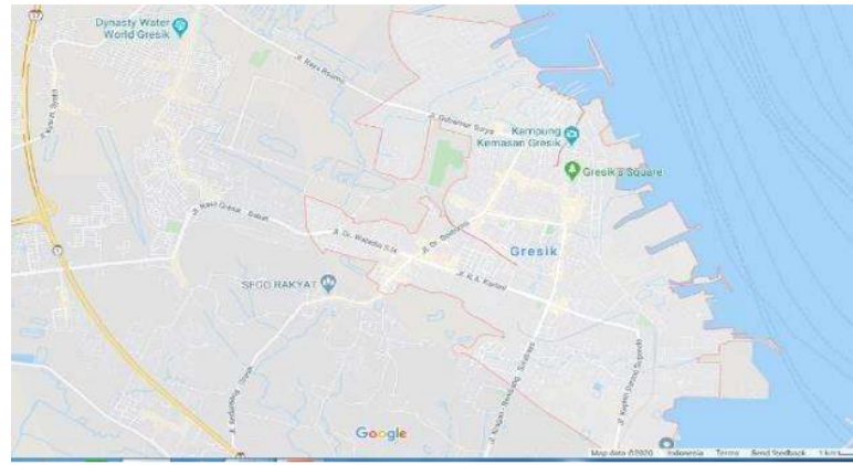
Gambar I. 1 Peta Lokasi Kabupaten Gresik
