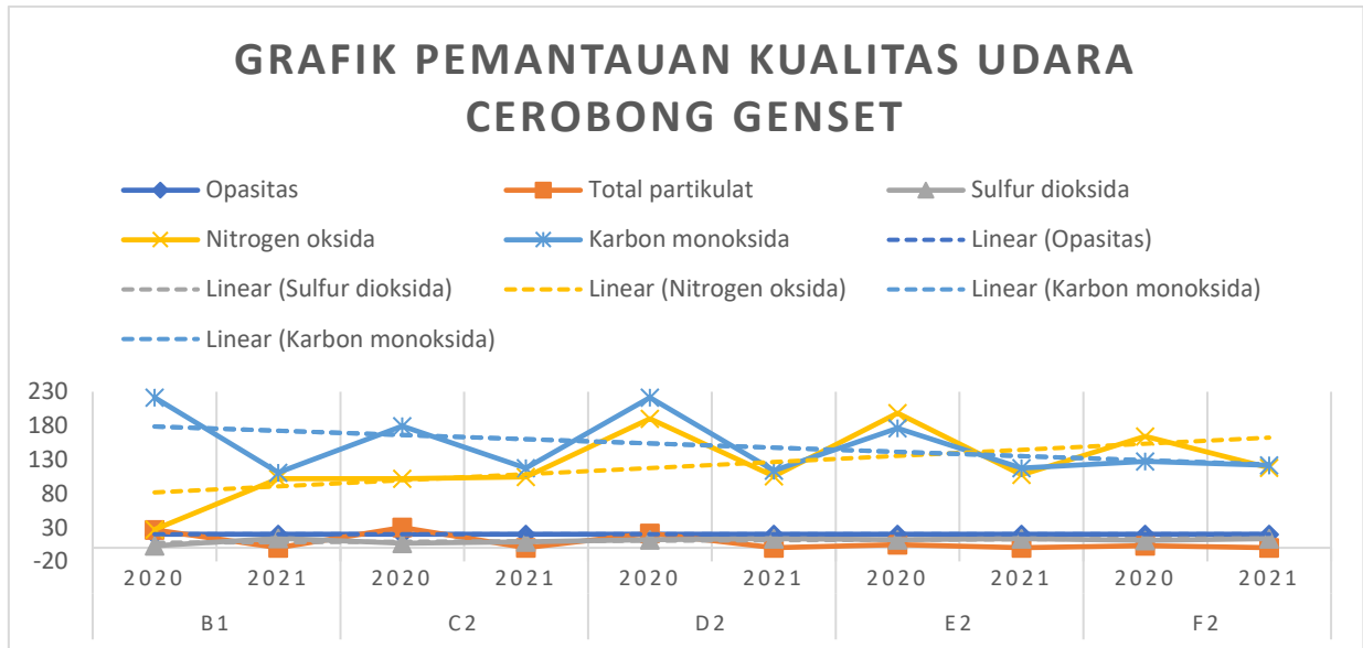
Gambar 4. Grafik Pengukuran Pemantauan Kualitas Udara Cerobong Genset
