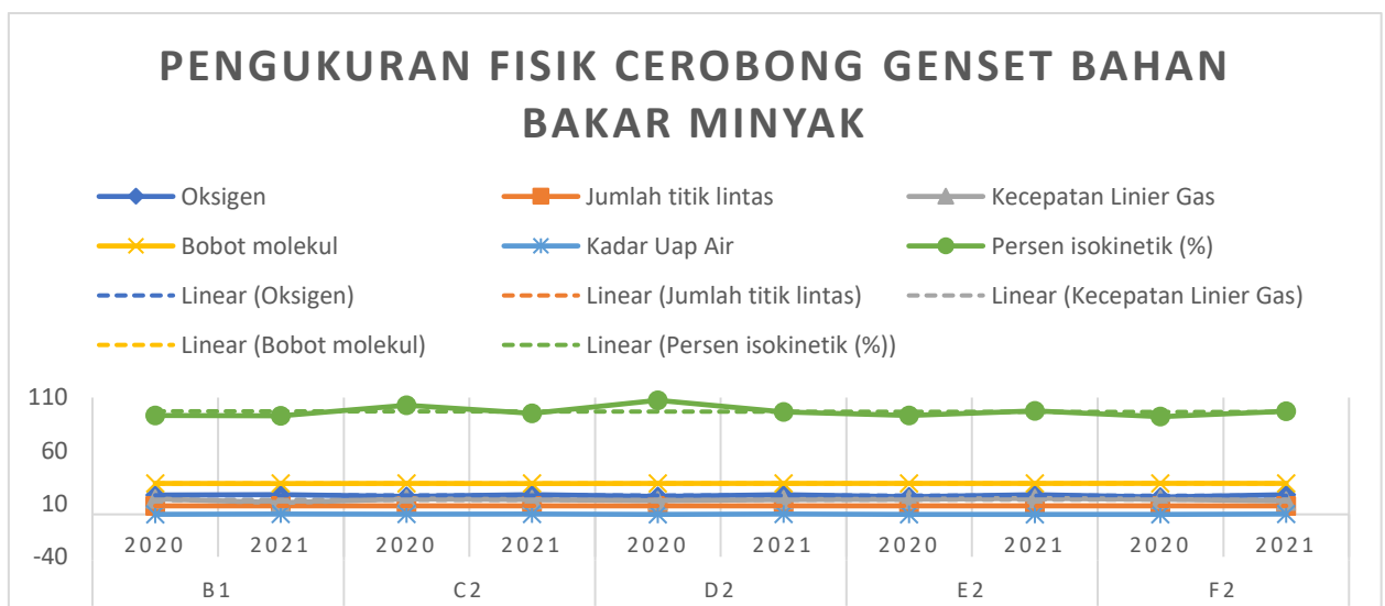
Gambar 3. Grafik Pengukuran Fisik Cerobong Genset Bahan Bakar Minyak
