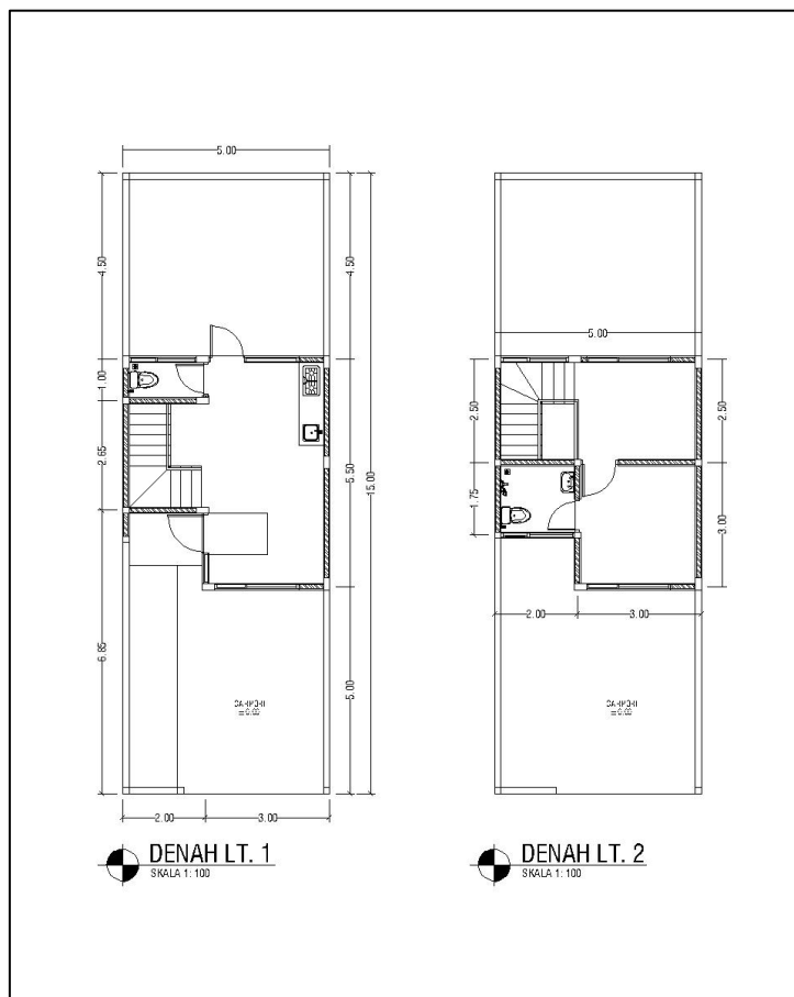
Alternatif Denah Rumah Milenial Type 50/75
