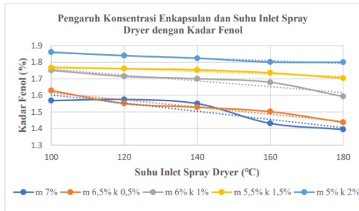
Gambar 6. Pengaruh Konsentrasi Enkapsulan dan Suhu Inlet Spray Dryer dengan Kadar Fenol
