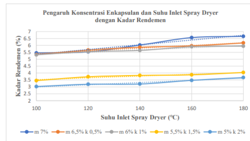
Gambar 4. Pengaruh Konsentrasi Enkapsulan dan Suhu Inlet Spray Dryer dengan Kadar Rendemen
