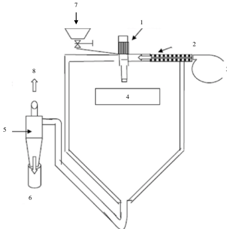
Gambar 1. Rangkaian Spray Dryer
