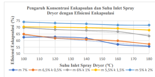
Gambar 7. Pengaruh Konsentrasi Enkapsulan dan Suhu Inlet Spray Dryer dengan Efisiensi Enkapsulasi
