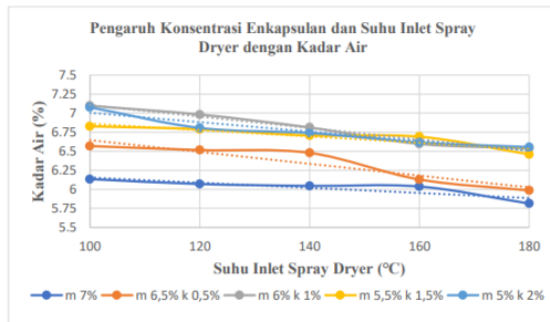
Gambar 5. Pengaruh Konsentrasi Enkapsulan dan Suhu Inlet Spray Dryer dengan Kadar Air
