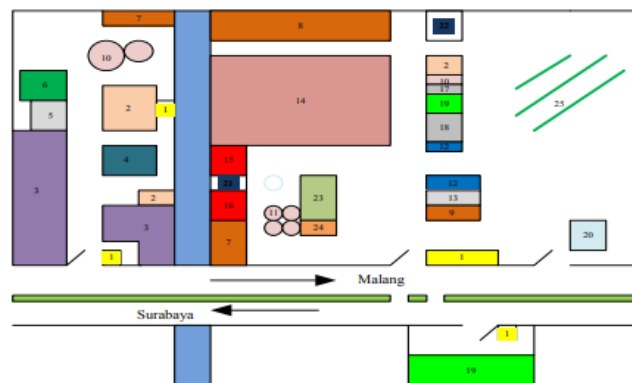
Gambar II.2 Tata Letak PT Pabrik Gula Candi Baru
