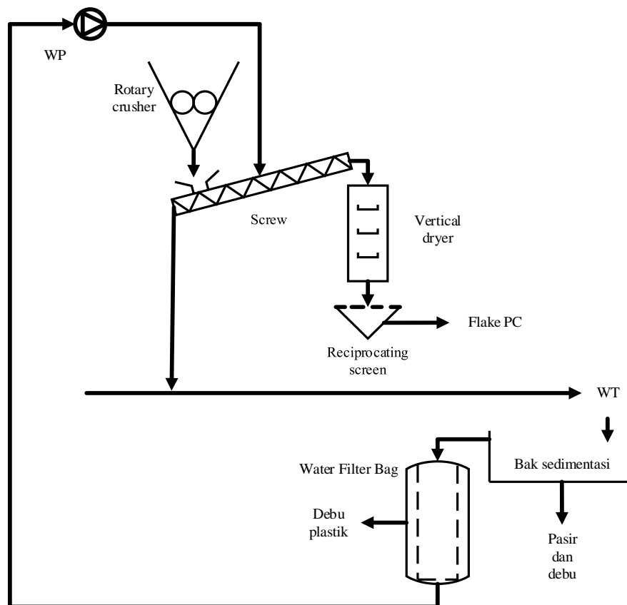
Gambar II. 2 Flowchart proses pengolahan limbah yang diusulkan
