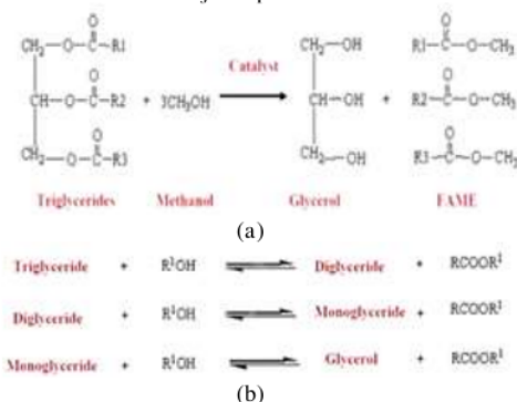
Gambar 3. (a) Reaksi transesterifikasi secara umum, (b) mekanisme reaksi transesterifikasi diadopsi dari (Athar and Zaidi, 2020)
