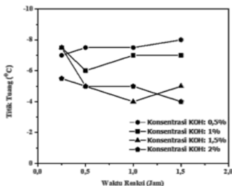
Gambar 5. Pengaruh konsentrasi KOH dan waktu reaksi terhadap titik tuang ( pour point ) biodiesel dari minyak biji kapuk
