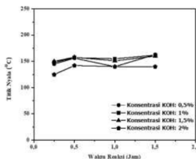
Gambar 4. Pengaruh konsentrasi KOH dan waktu reaksi terhadap titik nyala ( flash point ) biodiesel dari minyak biji kapuk
