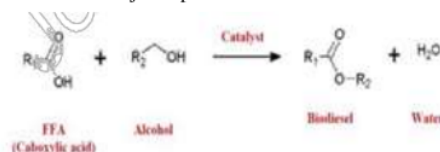
Gambar 2. Reaksi esterifikasi diadopsi dari (Athar and Zaidi, 2020)
