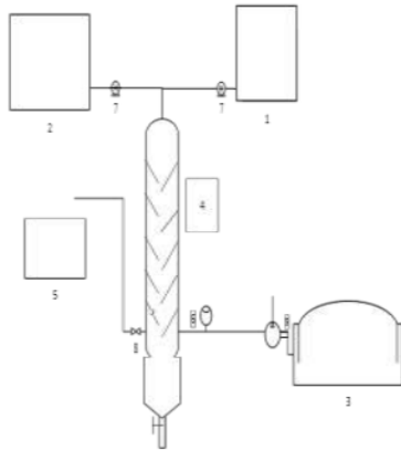
Gambar 1. Rangkaian Alat Reaktor Sekat Miring
