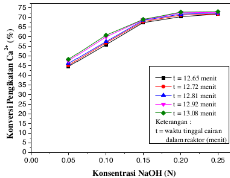
Gambar 3. Pengaruh Konsentrasi NaOH dan Waktu Tinggal terhadap Konversi Pengikatan Ca 2+
