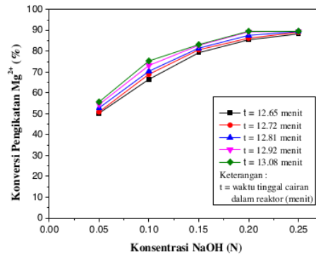
Gambar 4. Pengaruh Konsentrasi NaOH dan Waktu Tinggal terhadap Konversi Pengikatan \text{Mg}^{2+}
