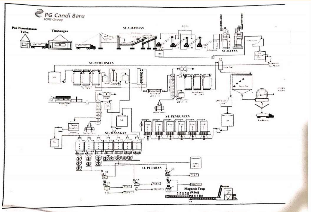
Gambar II.1. Flowsheet proses pengolahan gula di PT.PG Candi Baru
