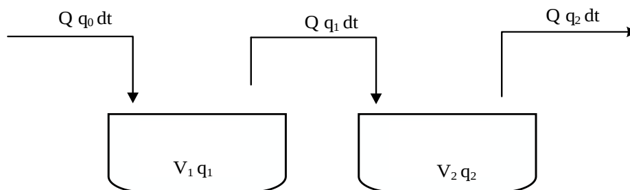
Gambar II.2 Skema Reaktor Tangki Alir Berpengaduk Pada Furnace
