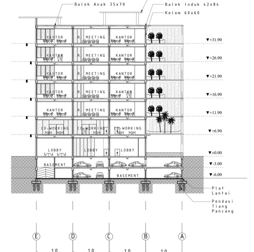
POTONGAN B-B
