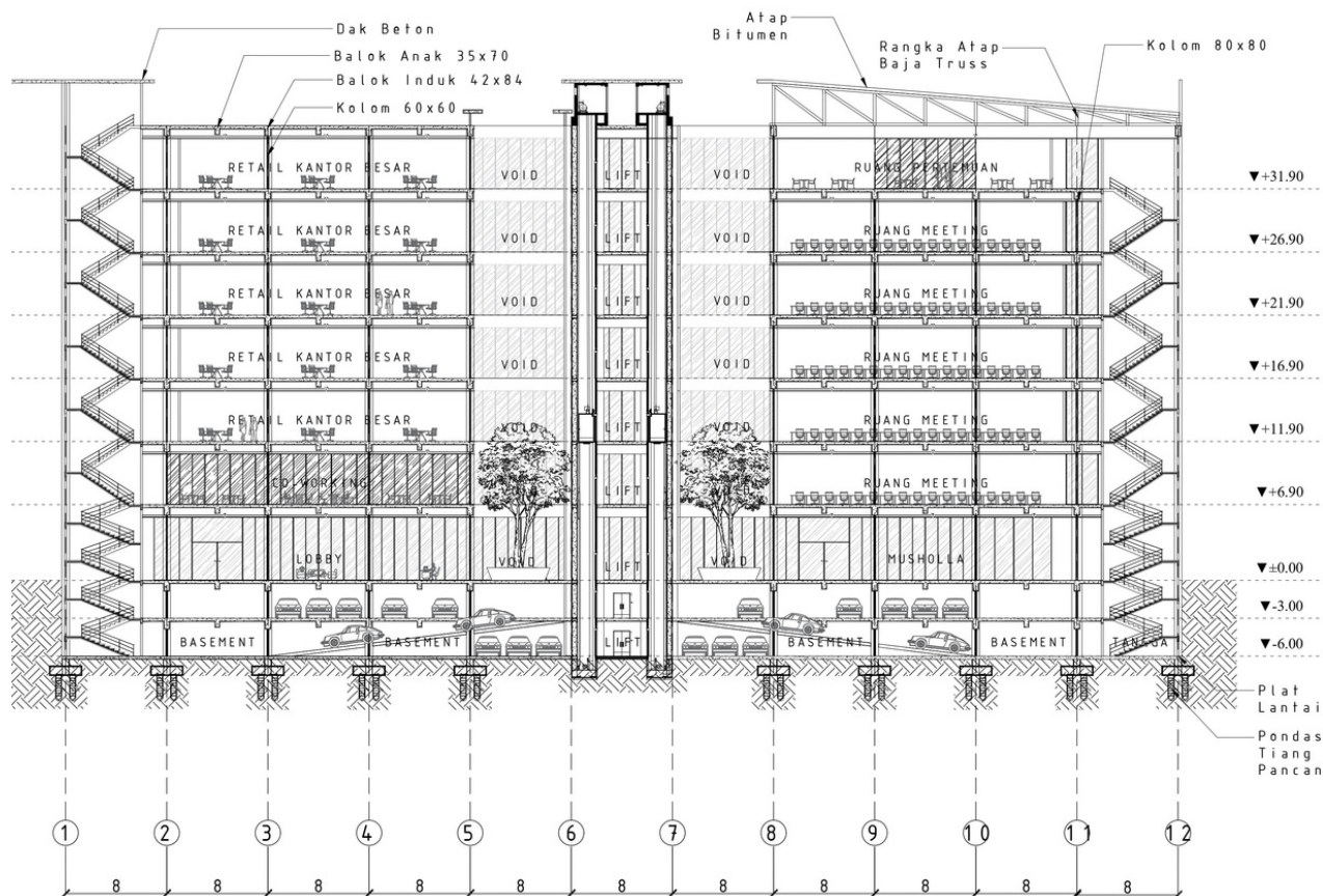
POTONGAN A-A
