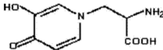
Gambar 2.1 Struktur mimosin
