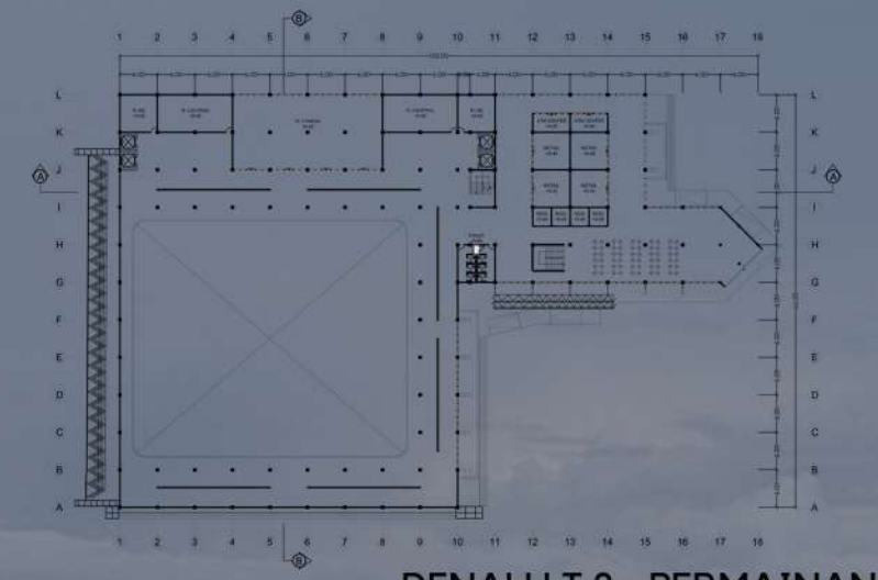
DENAH LT 2 - PERMAINAN
