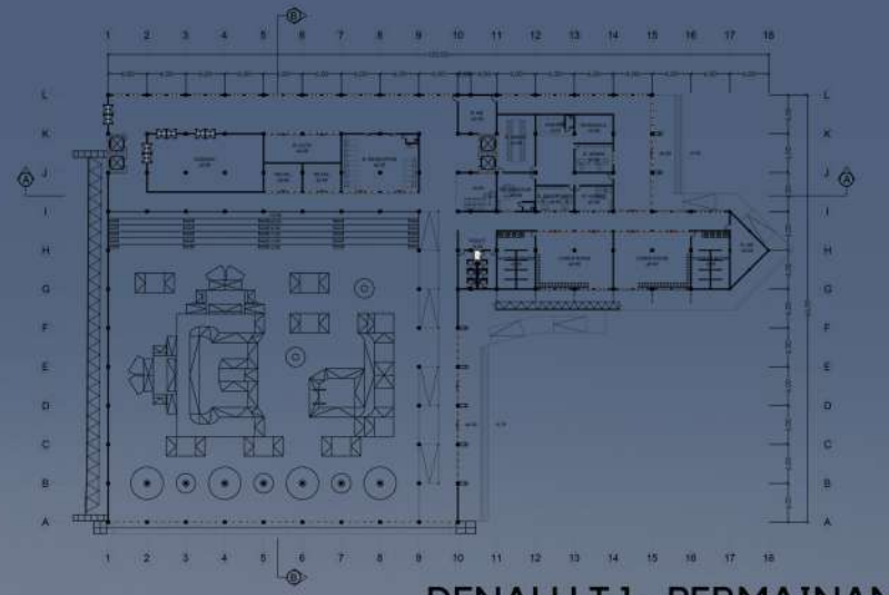
DENAH LT 1 - PERMAINAN
