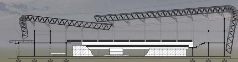
POTONGAN A - KOMPETISI
