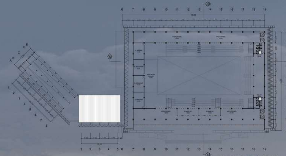
DENAH LT 2 - KOMPETISI
