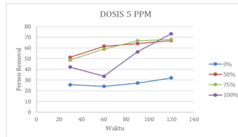
Gambar -10 Grafik Fluktuasi BOD (5ppm)
