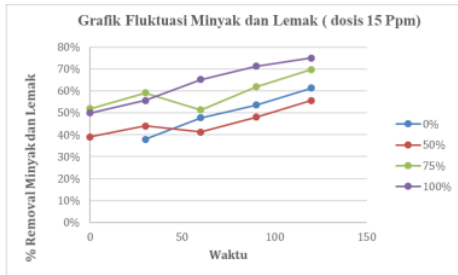
Gambar -8 Grafik Fluktuasi FOG (15 ppm)
