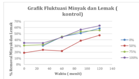
Gambar -5 Grafik Fluktuasi FOG (kontrol)
