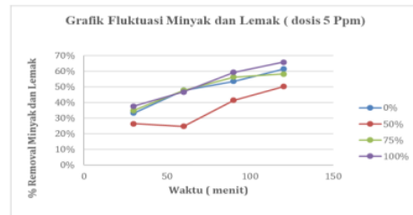
Gambar -6 Grafik Fluktuasi FOG (5ppm)
