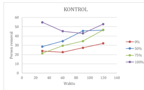
Gambar -9 Grafik Fluktuasi BOD (control)
