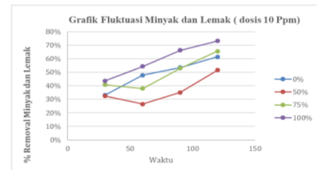
Gambar -7 Grafik Fluktuasi FOG (10ppm)
