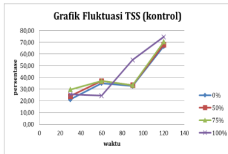
Gambar -1 Grafik Fluktuasi TSS (kontrol)
