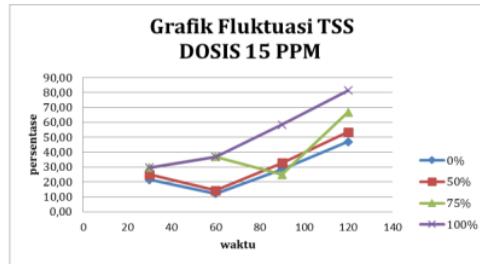
Gambar -4 Grafik Fluktuasi TSS 15ppm
