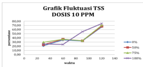
Gambar -3 Grafik Fluktuasi TSS 10ppm
