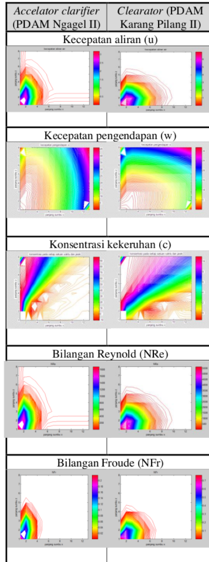
Gambar 2. Hasil Running Model HP2S dengan Bak Pengendap Jenis Sirkular
