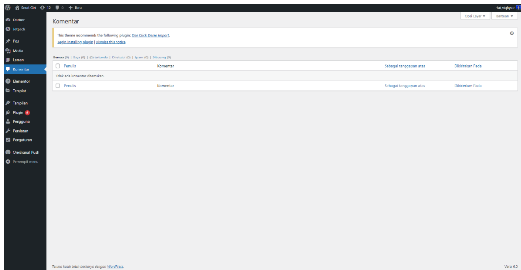
Gambar 2.7 Fitur Komentar
