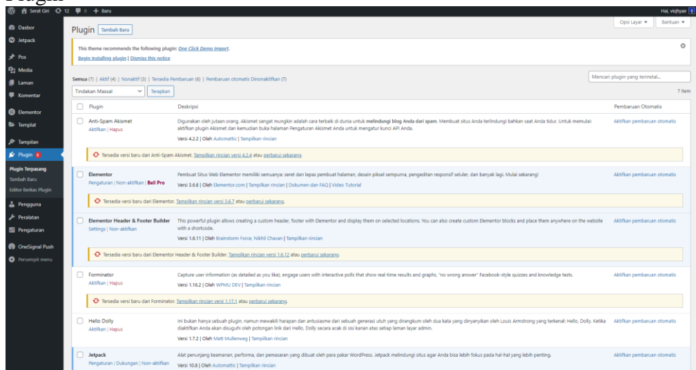
Gambar 2.9 Fitur Plugin
