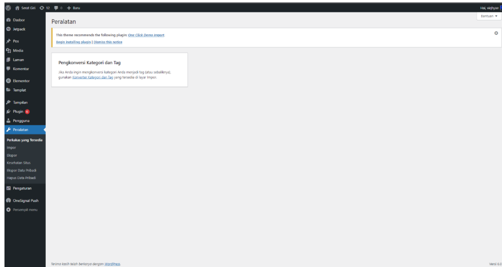
Gambar 2.11 Fitur Peralatan
