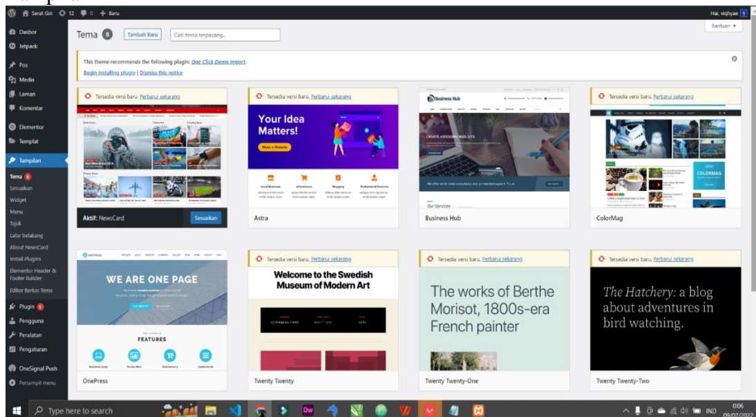
Gambar 2.8 Fitur Tampilan
