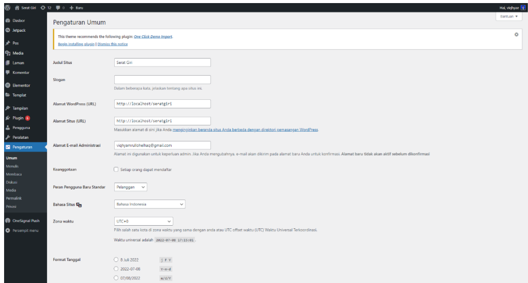
Gambar 2.12 Fitur Pengaturan
