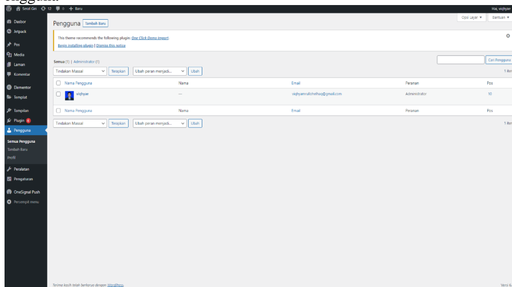
Gambar 2.10 Fitur Pengguna
