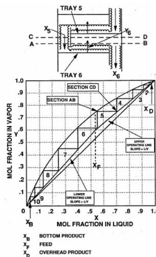
Gambar 8. Diagram Mc Cabe - Tiele
