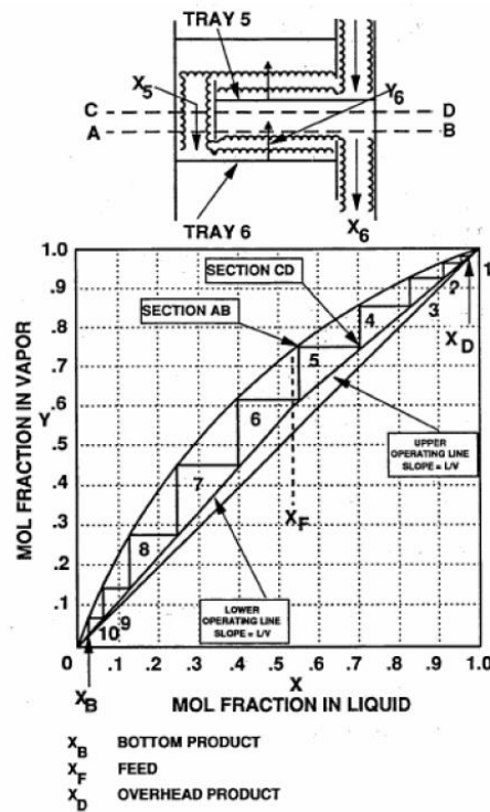
Gambar 21. Diagram McCabe-Tiele
