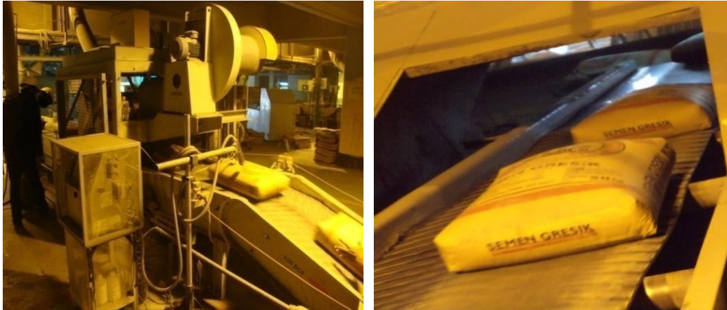
Gambar 3.18 Pengemasan ( Packer )
