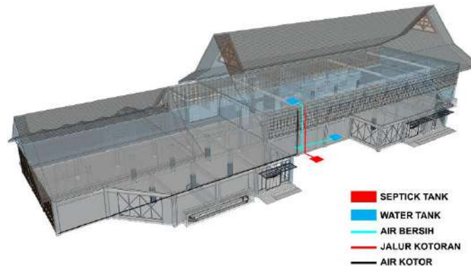
Gambar 6.14 Aplikasi Sistem Air Sumber : Ilustrasi Pribadi
