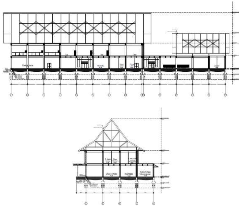
Gambar 6.10 Potongan Bangunan Sumber : Analisa Pribadi, 2023
