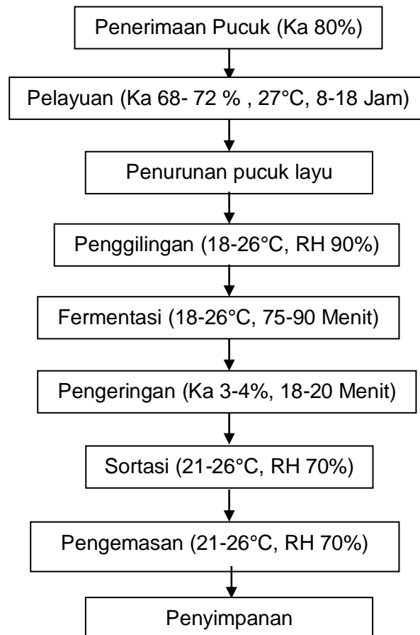
Gambar 2. Diagram Alir Proses Pengolahan Teh Hitam CTC di PTPN XII Kebun Wonosari (Sumber : PT Perkebunan Nusantara XII Kebun Wonosari, 2015)
