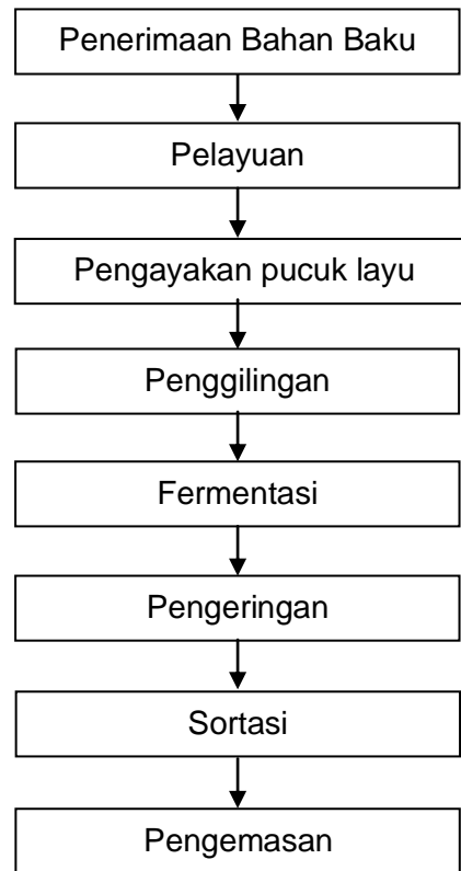
Gambar 1. Diagram Alir Proses Pengolahan Teh Hitam CTC (Sumber : Setyamidjaja,2000).
