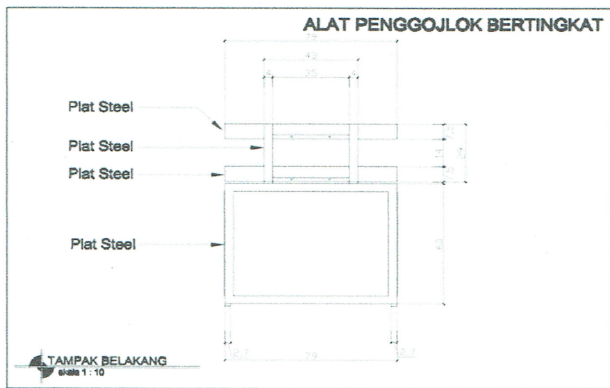
GAMBAR 3. TAMPAK BELAKANG, SAMPING KIRI DAN SAMPING KANAN ALAT PENGGOJLOK BERTINGKAT
