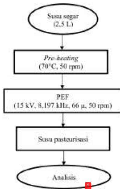
Gambar 1. Diagram alir proses pengolahan susu pasteurisasi
