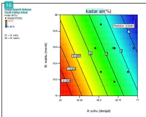
Gambar 7. Contour kadar air pektin pedada
