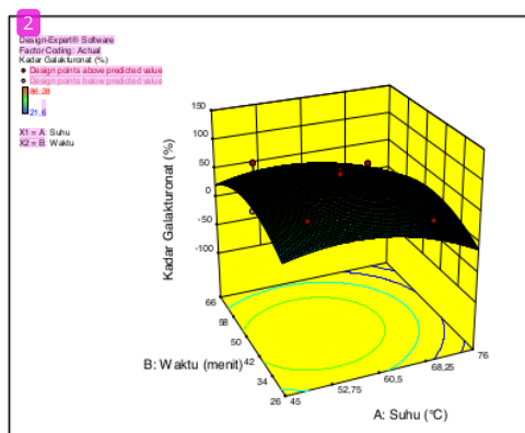
Gambar 4. 3D Surface Kadar Galakturonat Pektin Pedada
