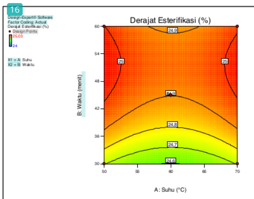
Gambar 5. Contour Derajat Esterifikasi Pektin Pedada
