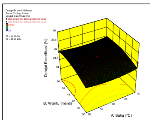
Gambar 6. 3D Surface Derajat Esterifikasi Pektin Pedada
