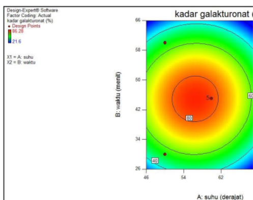
Gambar 3. Countour Kadar Galakturonat Pektin Pedada
