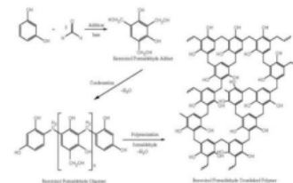
Gambar 4. Ikatan resorsinol-formaldehid
