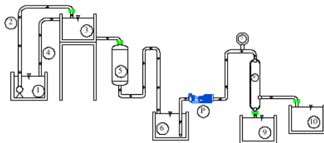
Gambar -1 Potongan Rangkaian Alat
