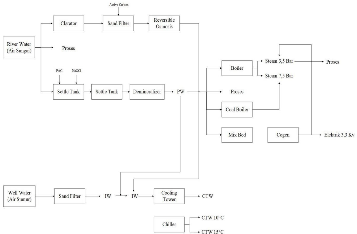
Gambar VI. 1 Diagram alir proses pengadaan air dan listrik ( PT. Ajinomoto Indonesia,2022 )
