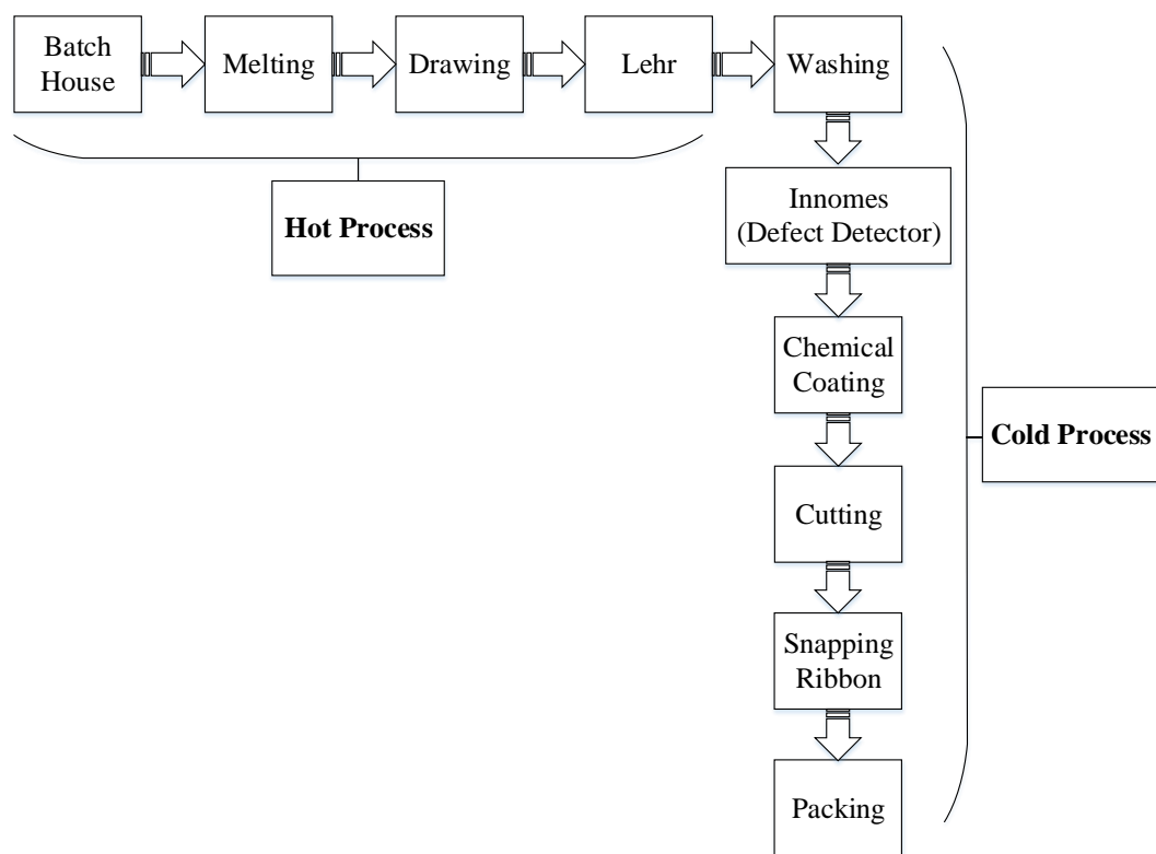
Gambar II.1 Alur Proses Produksi Kaca PT Asahimas Flat Glass Tbk Sidoarjo Factory
