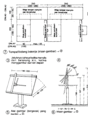
Gambar 1. Gambar tampak atas dan perspektif meja gambar
