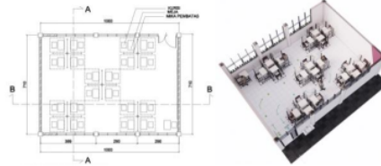
Gambar 11. Denah Ruang 3-1 tipe Round Table
