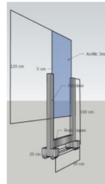
Gambar 17. Desain partisi pembatas
