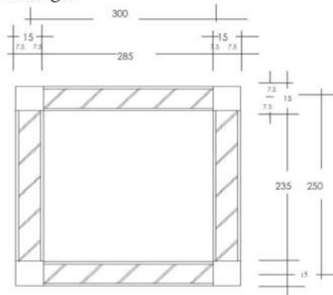
Gambar 12.12. notasi ukuran
