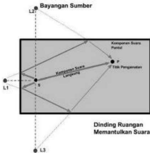
3 Gambar 10.14. Fenomena Suara dalam ruangan Sumber : http://peredamsuara.web.id/kinerja-peredam-suara/beranda/
