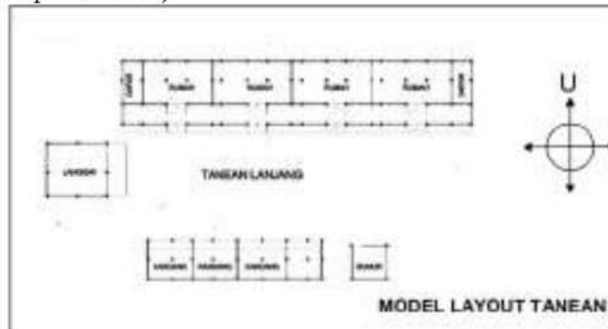
Gambar 2.35. Layout Rumah Tanean
