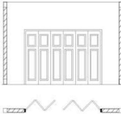
Gambar 12.19. tampak depan dan tampak atas pintu lipat
