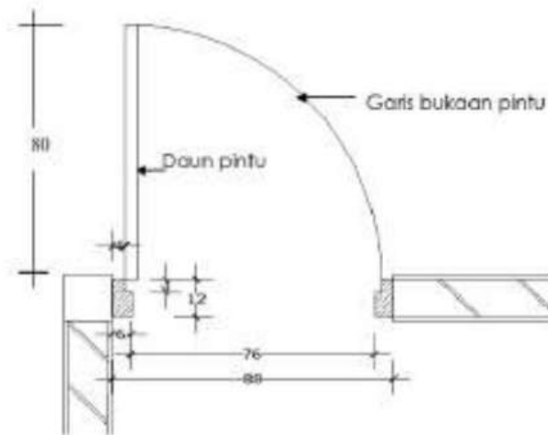
Gambar 12.16.detail pintu
