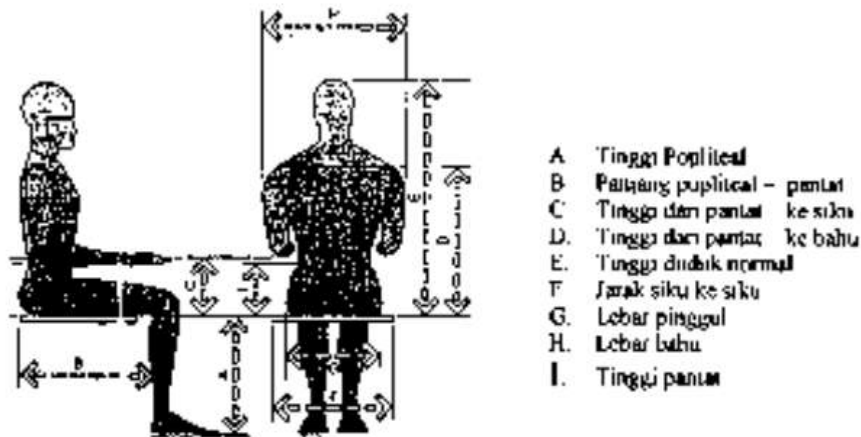
Gambar 5.4. Anthropometri pokok yang dibutuhkan untuk desain tempat duduk Sumber : Kusuma L,2003
