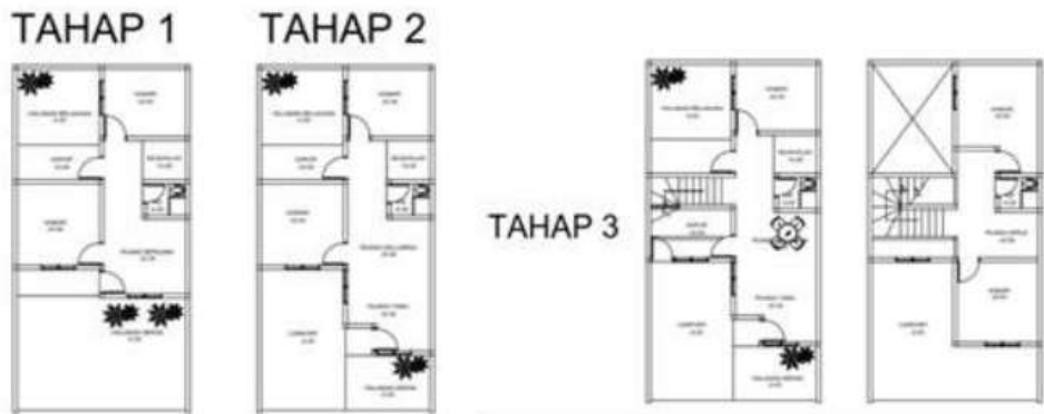
Gambar 6.16. Denah tahapan perubahan rumah tumbuh tipe 21 m2 Sumber : Agustin D,2019
