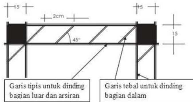
Gambar 12.13. detail teknik penggambaran dinding
