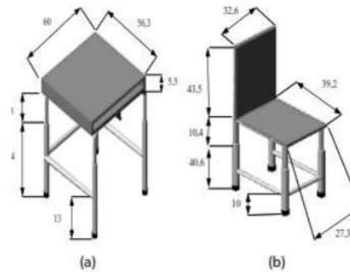
2 Gambar 5.6. (a) merupakan gambar detail hasil redesain meja dan Gambar 2 (b) merupakan gambar detail hasil redesain kursi.
