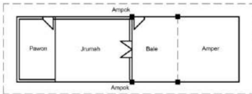
Gambar 2.23. Denah Rumah Osing Sumber : Perbup no 11 tahun 2019
