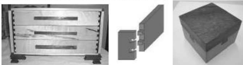
Gambar 2.1. sambungan dovetail (ekor burung)
