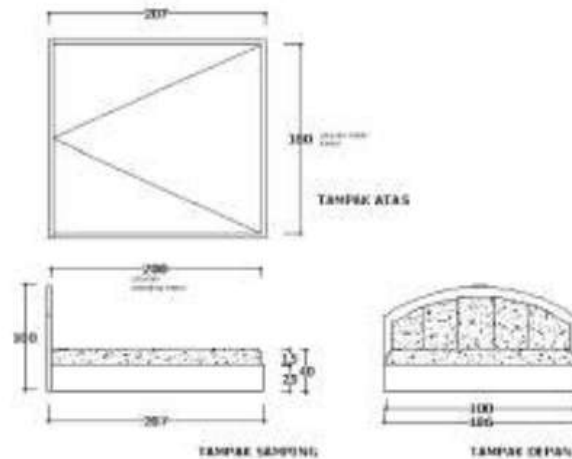
Gambar 12.26.detail tempat tidur
