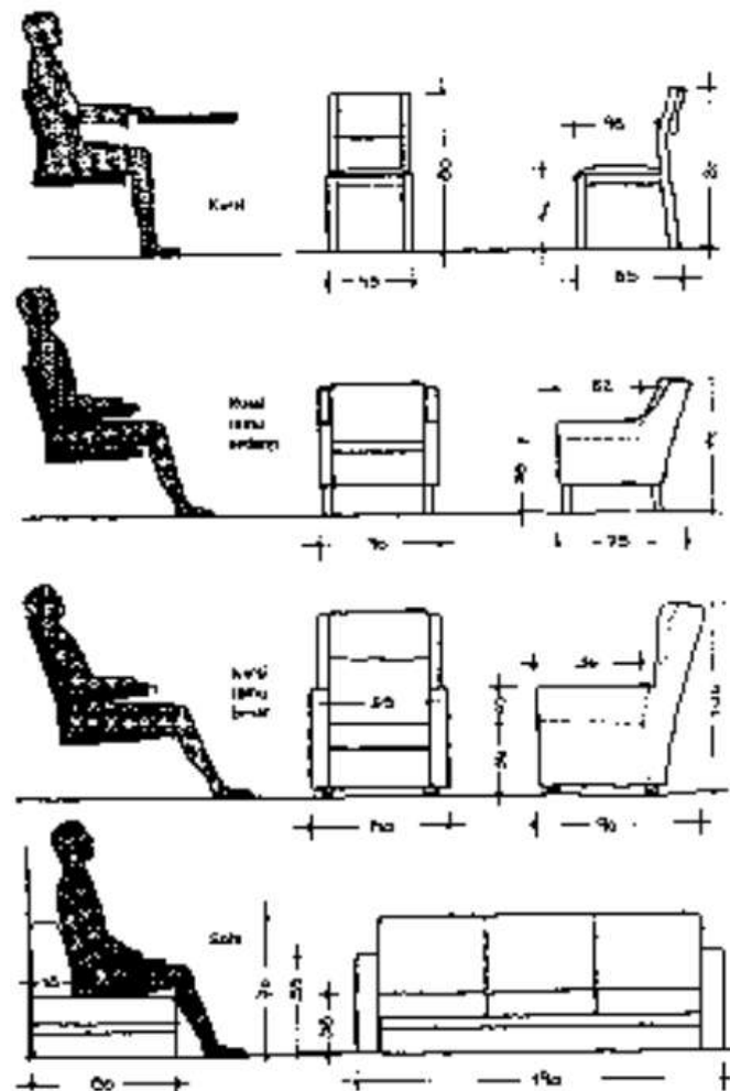
Gambar 7.2. Bentuk macam macam kursi Sumber : Suptandar J, 1999
