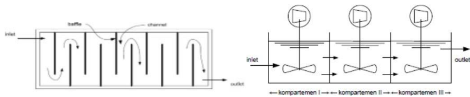
Gambar 2. 3 Pengadukan Lambat Secara Mekanis dan Secara Hidraulis
