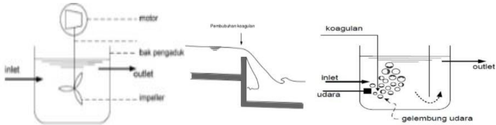
Gambar 2. 2 Pengadukan Mekanis, Pengadukan Hidraulis dan Pengadukan Pneumatis
