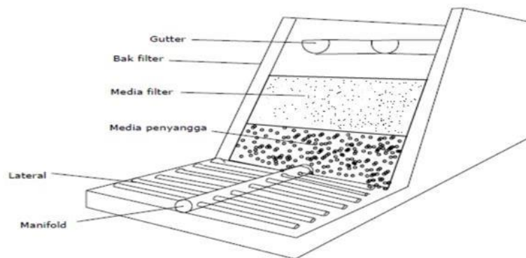
Gambar 2. 7 Struktur Filter Pasir Cepat
