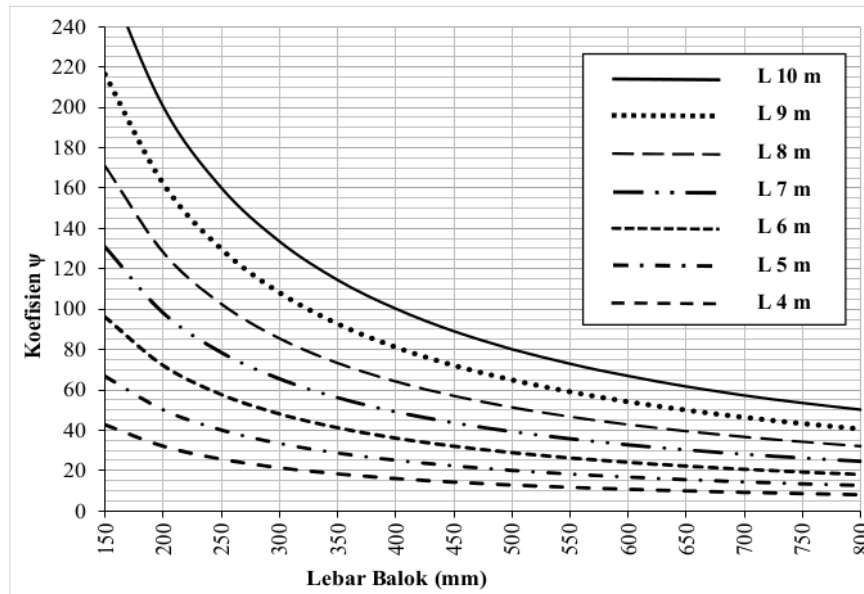
Gambar 7. Grafik perbandingan antara lebar balok dengan koefisien \psi untuk berbagai variasi dimensi dan bentang jembatan.
