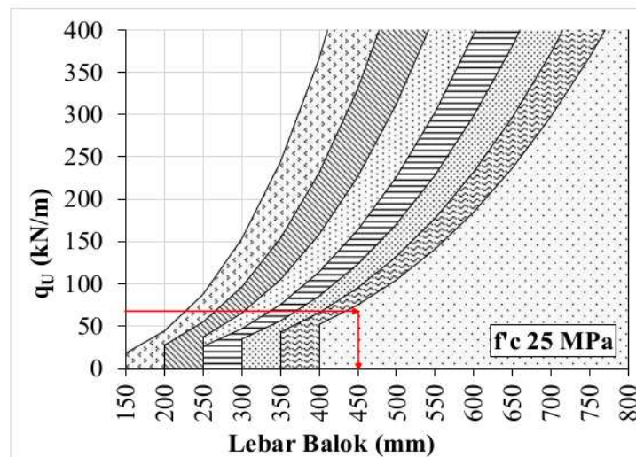
Gambar 8. Cara menentukan lebar balok yang diperlukan.
