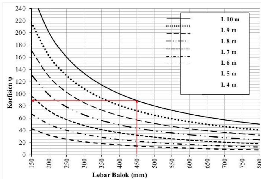
Gambar 9. Cara menentukan nilai koefisien \psi
